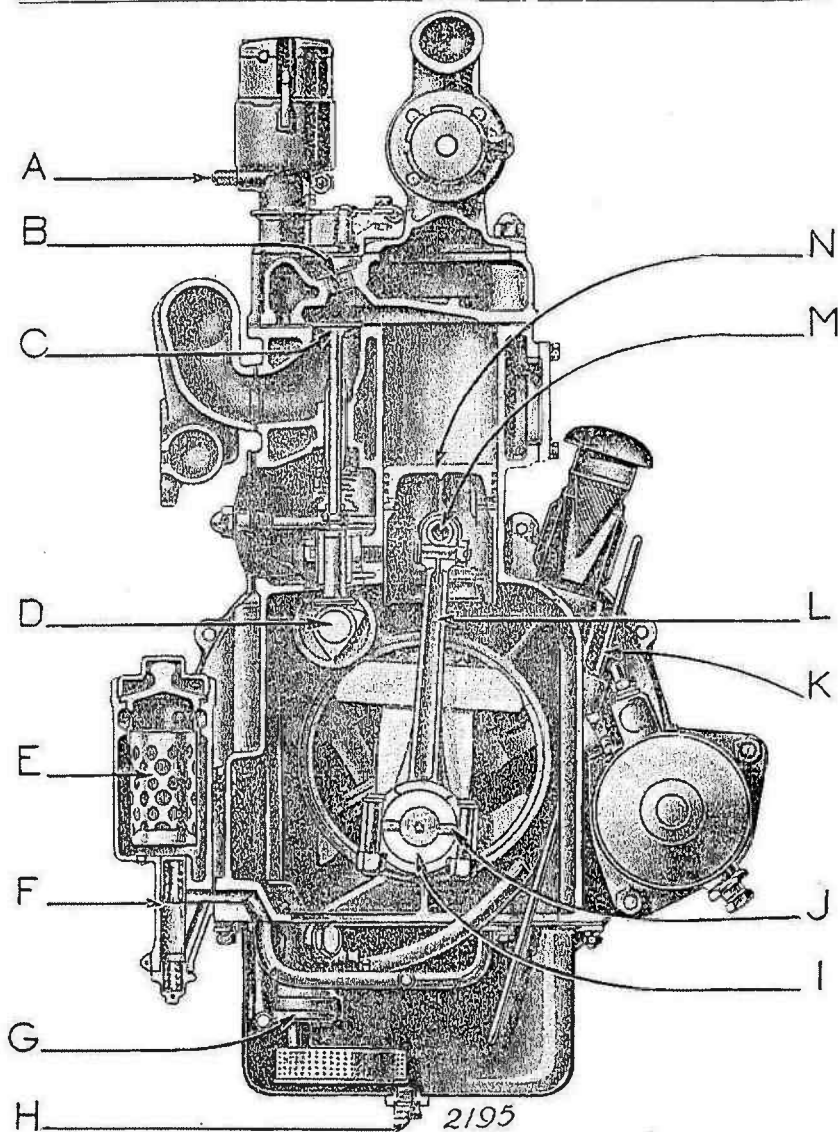
Fig. 5. — Coupe transversale du moteur.
