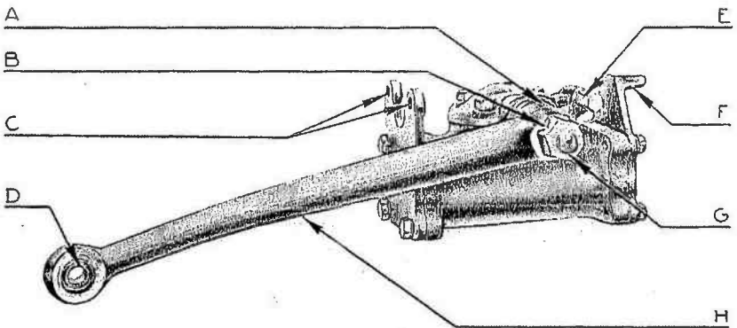
Fig. 10. — Amortisseur hydraulique.
