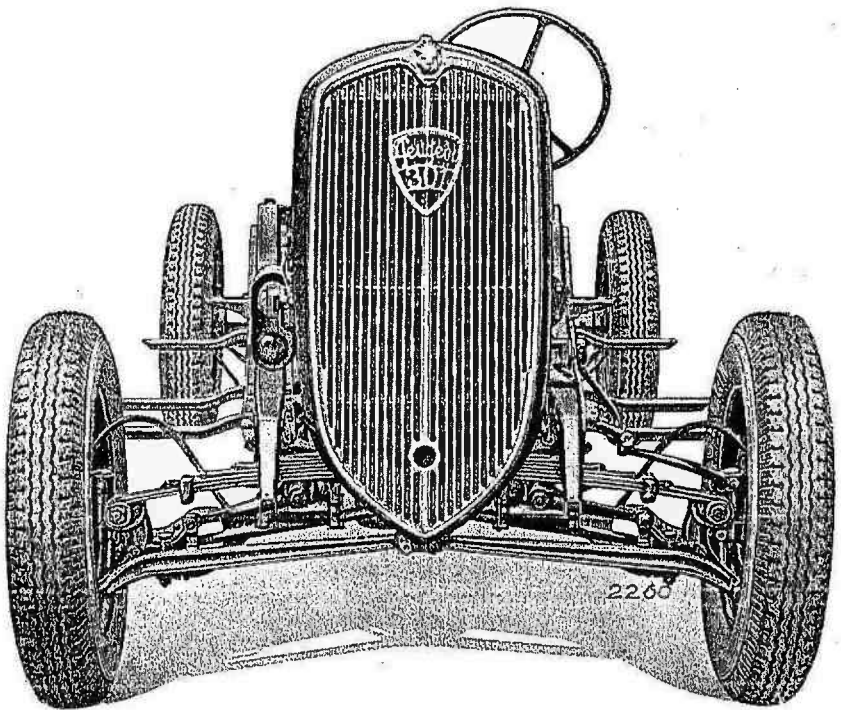
Fig. 1. — Vue de face du châssis.
