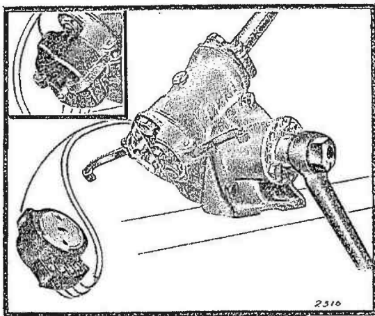
Fig. 39. — Commutateur démonté.
