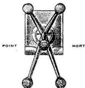
Fig. 41. — Schéma des positions du levier des vitesses des boîtes "standard" synchronisées.
