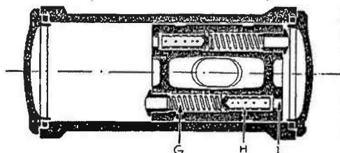
Fig. 12. — Coupe schématique montrant le fonctionnement des amortisseurs.
