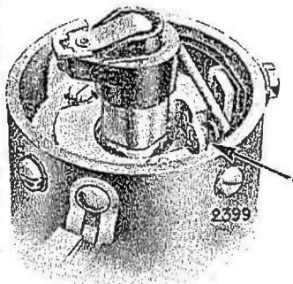
Fig. 35. Écartement des contacts.
