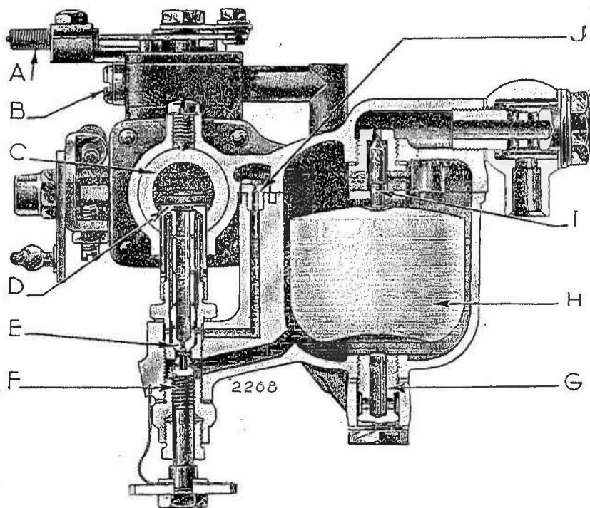
Fig. 14. — Fausse coupe montrant les organes intérieurs du carburateur.
