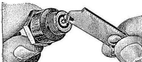
Fig. 35. Outil permettant de régler l'écartement des pointes sans risquer de casser l'isolant.
