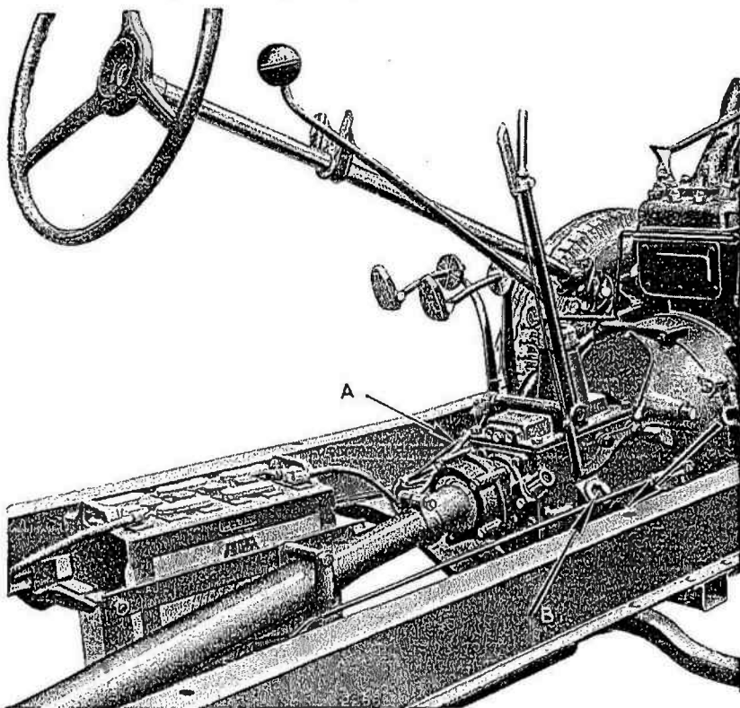
Fig. 28. — Vue de la boîte de vitesses et du joint de cardan. A) Graisseur du joint de cardan; B) Bouchon de remplissage de la boîte de vitesses formant niveau d'huile; C) Bouchon de vidange.
