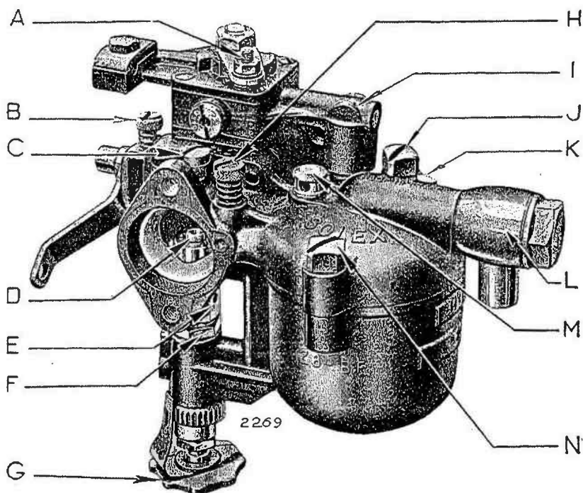
Fig. 15. — Carburateur.
