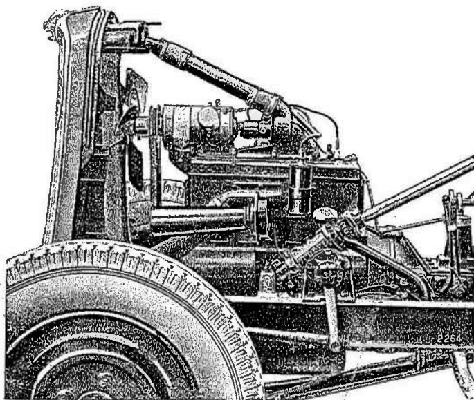
Fig. 27. — Vue latérale gauche du moteur.
