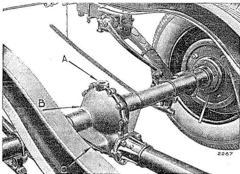
Fig. 29. — Graissage du pont arrière : A) Bouchon de remplissage ; B) Bouchon de niveau ; C) Bouchon de vidange.
