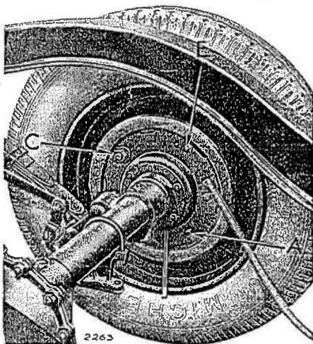
Fig. 23. — Réglage des freins arrière.
