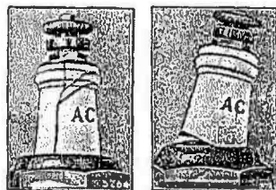
Fig. 36. Cassures provoquées par choc ou mauvaise manutention.
