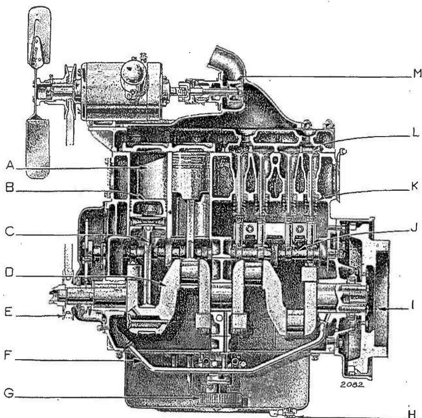
Fig. 4. — Coupe longitudinale du moteur.
