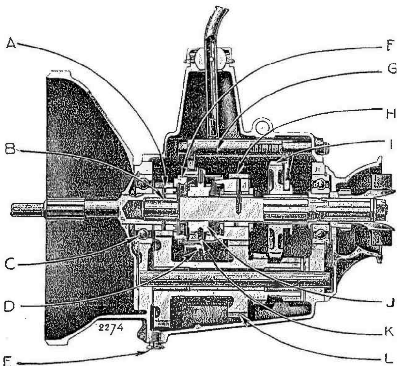
Fig. 7. — Coupe longitudinale de la boîte de vitesses.
