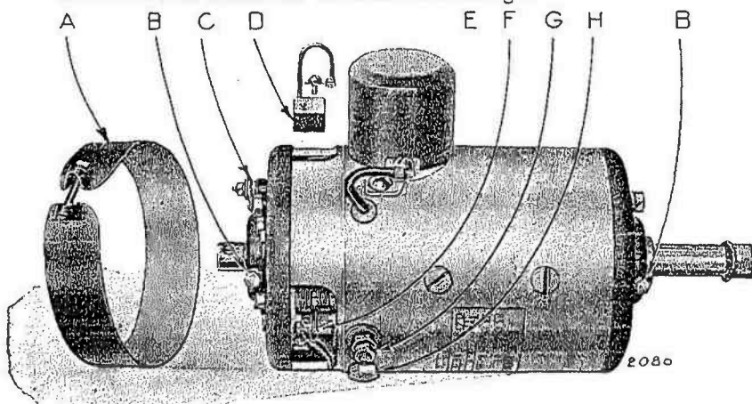
Fig. 37. — Vue de la dynamo avec sangle enlevée (nouvelle dynamo compound).
