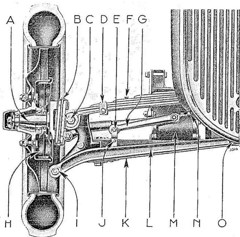
Fig. 9. — Coupe de l'essieu avant droit.
