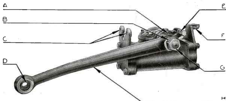
Fig. 10. — Amortisseur hydraulique.
