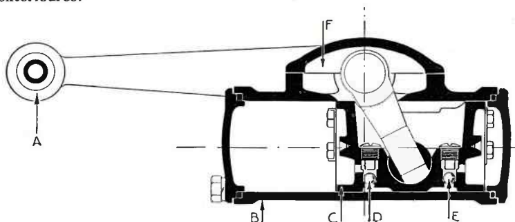
Fig. 11. — Coupe longitudinale.
