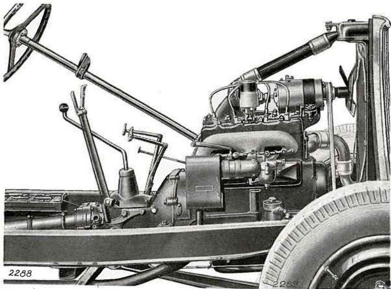
Fig. 16. — Vue latérale droite du moteur
